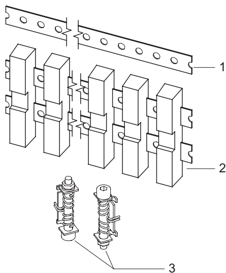
Рис. 34 Анодная лента
