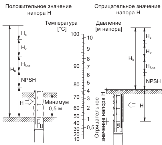
Рис. 20 Глубина установки
