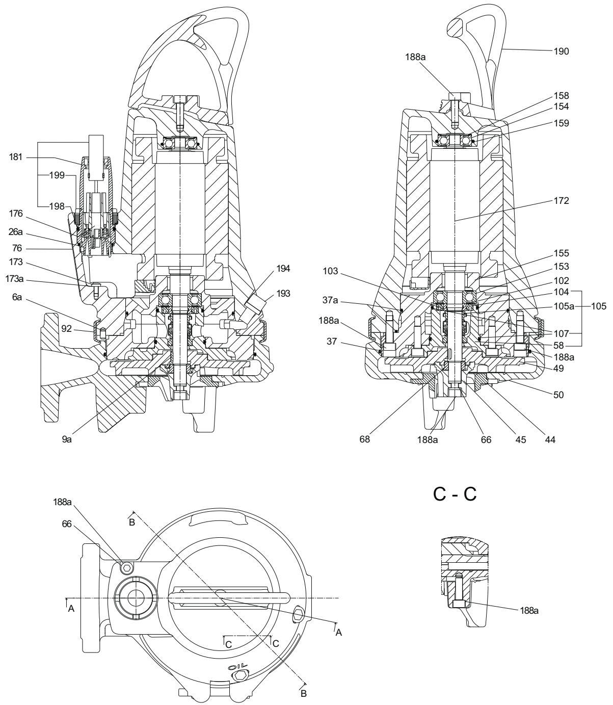
Рис. 8 Чертеж насоса SEG в разрезе, 0,9, 1,2 и 1,5 кВт
