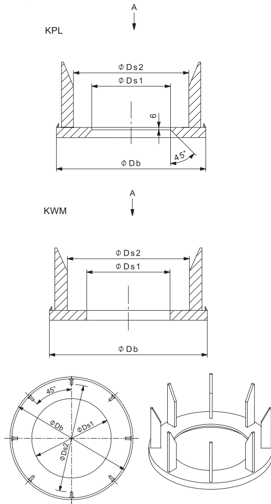
Рис. 28 Установочное кольцо
