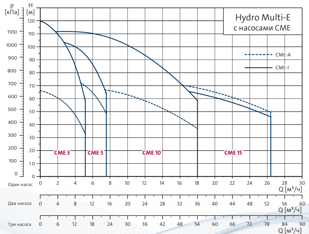
Рабочие характеристики Hydro Multi-E с насосами СМЕ
