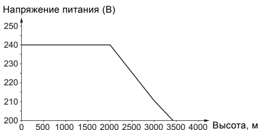
Рис. 35 Напряжение питания для однофазного электродвигателя в зависимости от высоты над уровнем моря
