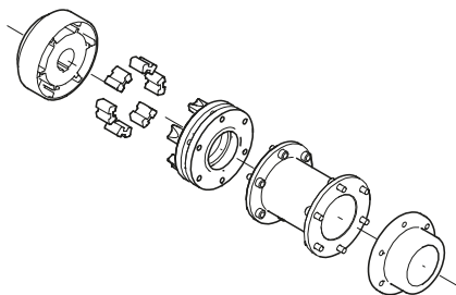
Рис. 24 Муфта с проставкой
