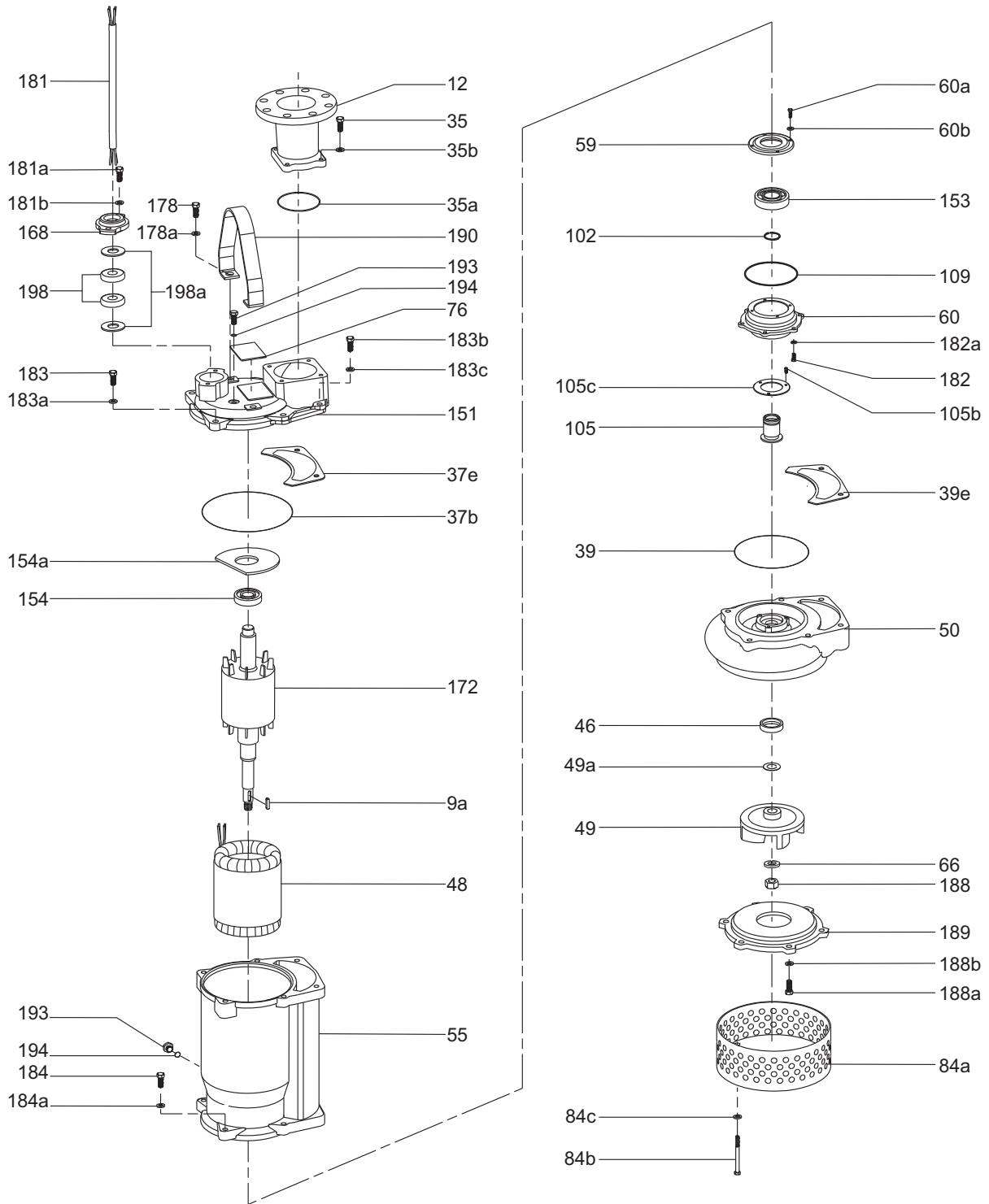
Рис. 7 Детализовка DWK.O.6.80.15, DWK.O.6.80.22, DWK.O.10.80.37 и DWK.O.10.100.37
